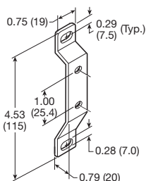
T-Bracket
