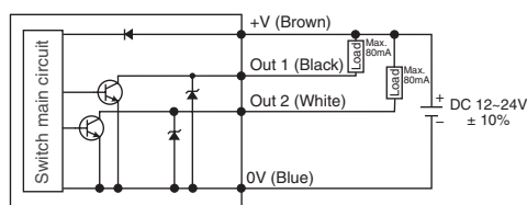
NPN Output
